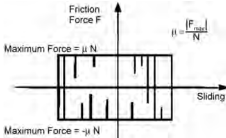
شکل ۲. عملکرد دینامیکی اتصال لوبیایی.
