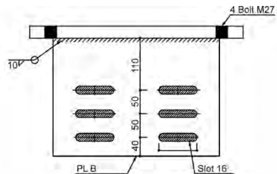
الف) قطعه متحرک میراگر عضو "T" شکل
