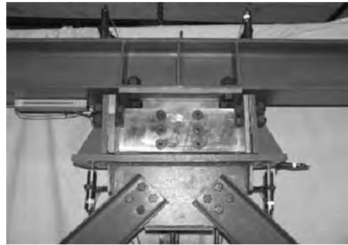
شکل ۸. موقعیت میراگر اصطکاکی در قاب.
